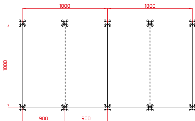
Dopuszczalne siły w podporach dla danej grubości stropu (Maksymalna powierzchnia wpływu na podporę A_2 = 1,62 \text{ m}^2 – płyty 0,9 \text{ m} \times 1,8 \text{ m} )
