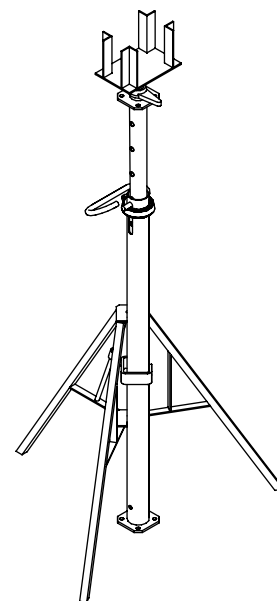
Schemat montażu podpory w trójnóg
