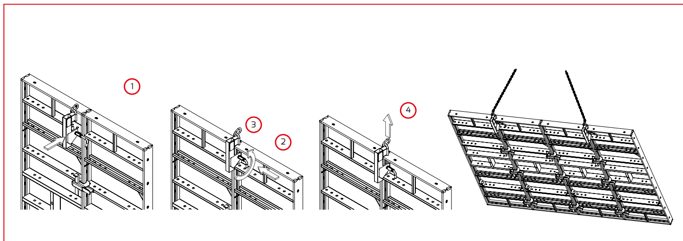
Hak transportowy - zastosowanie
