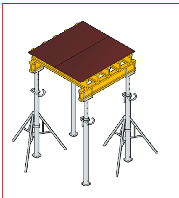
Zastosowanie trójnoгу - schemat
