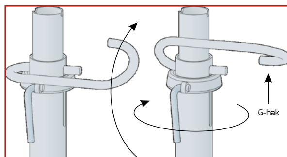
Kolejność postępowania przy odciążaniu podpory przy użyciu G-haka
