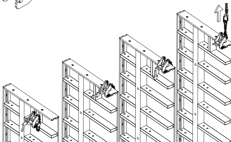
Zawiesie transportowe - przykład montażu
